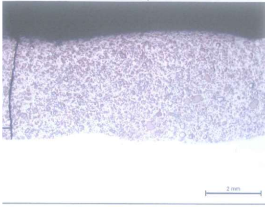
Påsvejst lag tætpakket med wolfram karbider.
