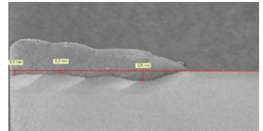
Stort set ingen ind-brænding i grundmaterialet.
